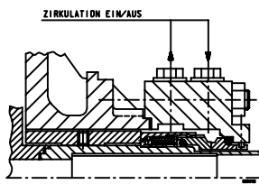
Gleitringdichtung mit luftgekühltem Wärmetauscher
