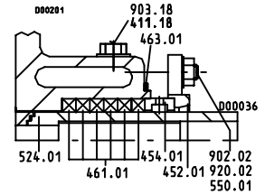
Packungsausführung gekühlt
