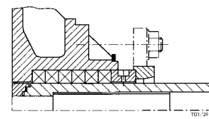
Packungsausführung ungekühlt Zusatzbezeichnung "x"
