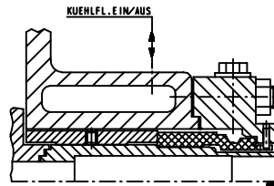
Gleitringdichtung einfachwirkend, intensiv gekühlt
