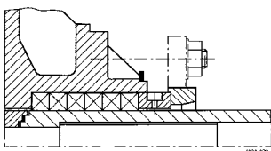
Stopfbuchspackung ungekühlt
