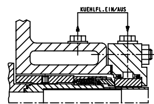
Gleitringdichtung einfachwirkend, intensiv gekühlt mit Gegenringkühlung
