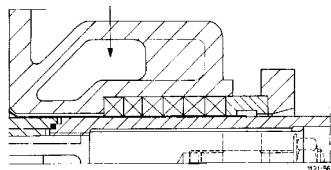
Stopfbuchspackung gekühlt
